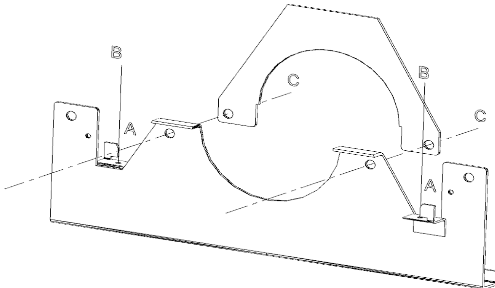
RYS. 6. Wspornik do promiennika SBT wersja „I”
