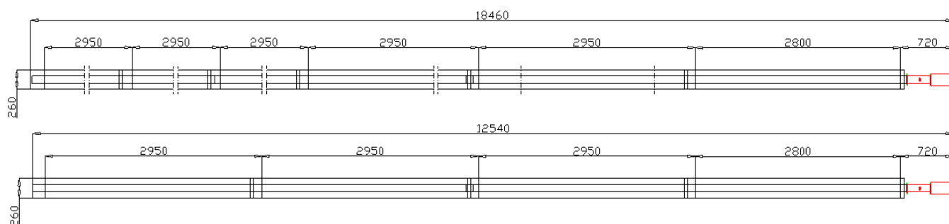
RYS. 2 Wymiary palnika i zmontowanych urządzeń SBT w wersji „U”
