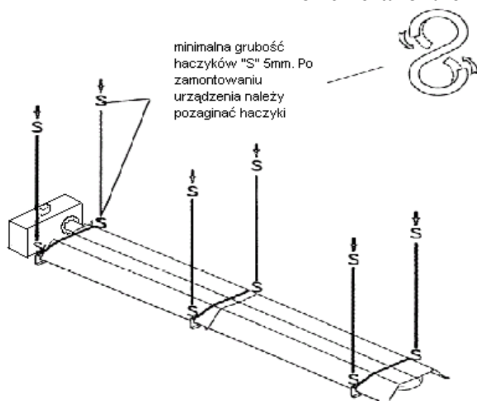
RYS. 17. Montaż promiennika na łańcuchach.
