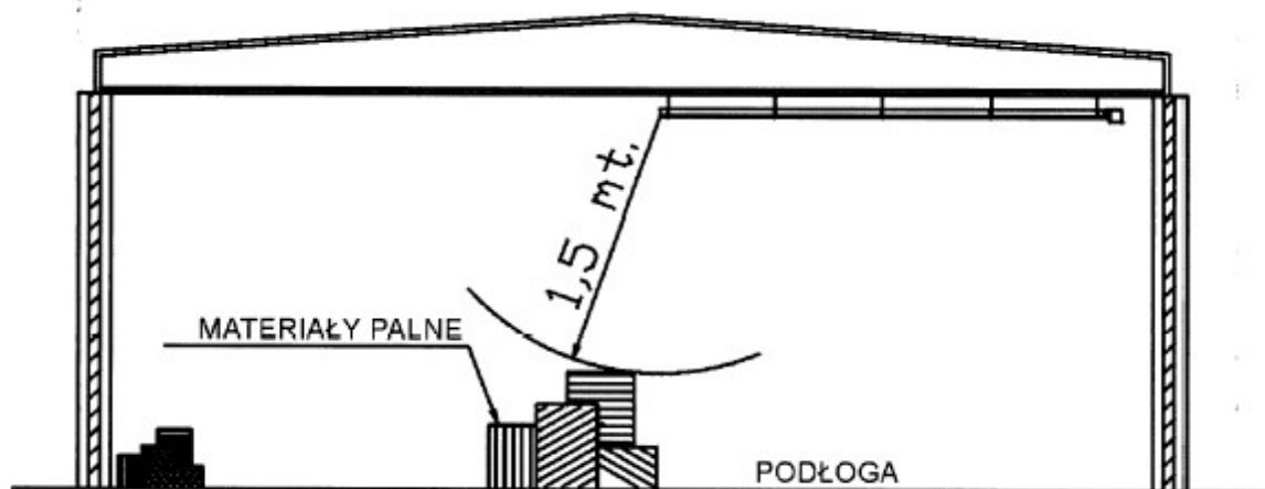
RYS. 12. Odległość od materiałów palnych
