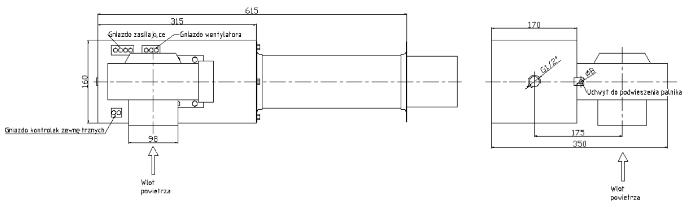
S. 4. Podstawowe wymiary palnika
