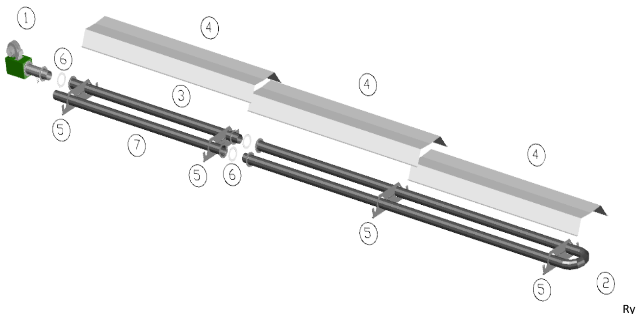
s. 1 Zestaw SUN-BEAM TUBES w wersji „U” / „I”
