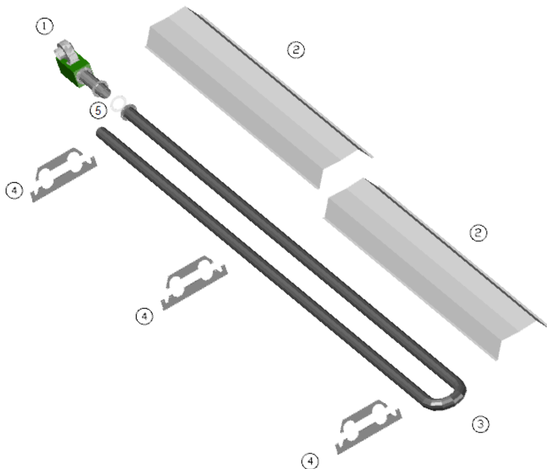
RYS. 7. Widok promiennika SBT 6U .
